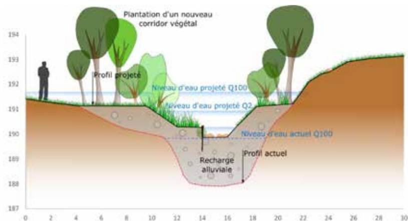
Profil projeté de la rivière la Mâtre
